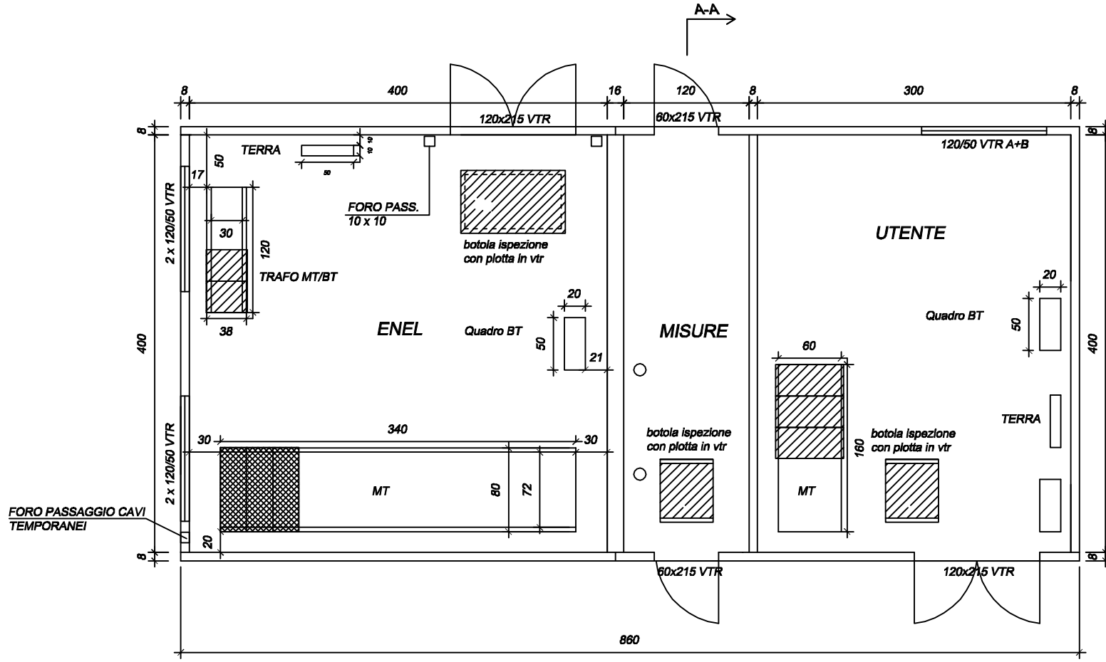
PIANTA CABINA
