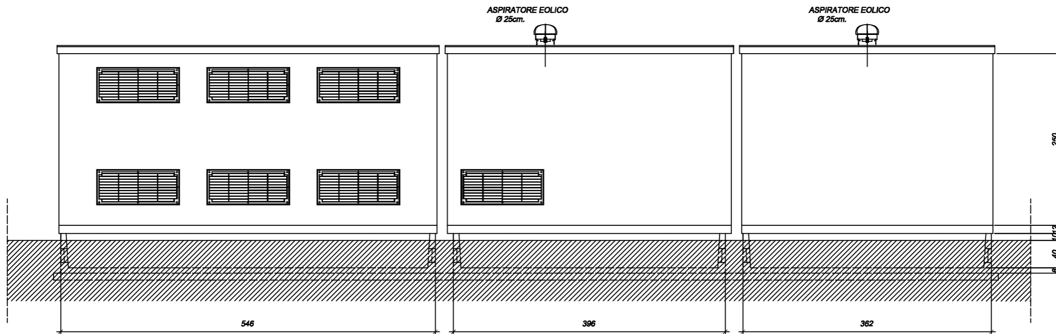
PROSPETTO POSTERIORE (A) - Rapp. 1:50
